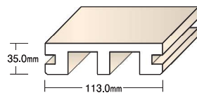
引違い戸用上部枠
