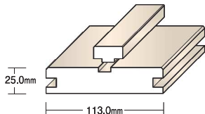
差込型内部ドア枠
