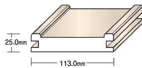
引き戸用縦枠(左右兼用)
