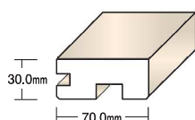
差込型折戸用上部枠 RC201-19 \ell=1900\text{mm} ¥6,600
