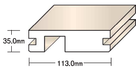
片引き戸用上部枠
