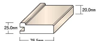
片引き戸用 戸当
