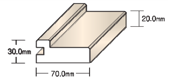
折戸用上レール (別途)
