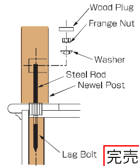
ニューエルポストファスナー LJ-3070 ¥6,000
