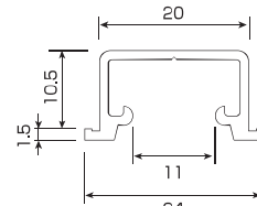
折戸用上レール
