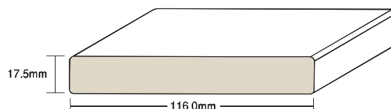
完売 MDF S4Sボード MD1X5 ℓ=12'・3660mm ¥3,900
