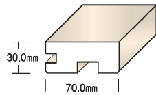
折戸用上レール (別途)
