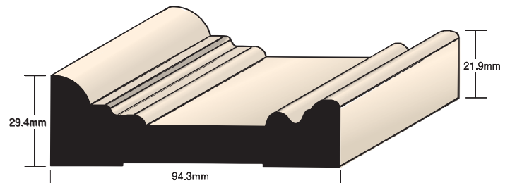
ケーシング / アーキトレイブ H5000 ℓ=10・3050 ㊦ ¥6,800
