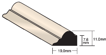
パネルモールド H703 ℓ=10'-3050mm ¥1,600
