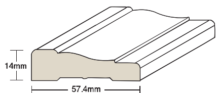
ケーシング MD356 ℓ=7'・2135mm ¥1,200 ℓ=12'・3660mm ¥2,200
