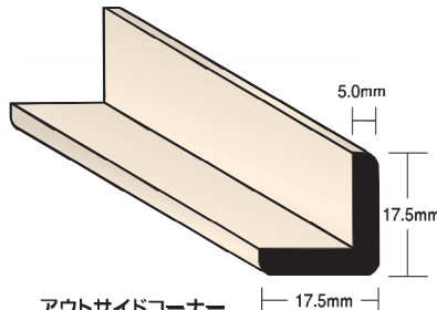
アウトサイドコーナー H3282 ℓ=12'-3660mm ¥2,800
