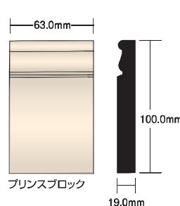
プリンスブロック HP3.5 ¥1,200
