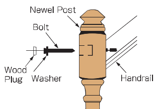
レールポストファスナー LJ-3078 ¥600
