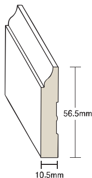
ベースボード MD625 ℓ=12'・3660 ㊦ ¥2,600
