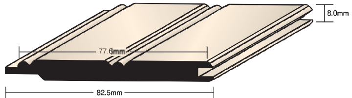
パネリング H216 板柎混合 ℓ=3'・890 ㎥ 15枚入 ¥7,900 8'・2440 ㎥ 15枚入 ¥33,000
