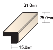
縦用 RC016-21 L=2150mm ¥3,100/本
