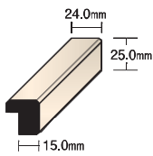
縦用 RC009-21 L=2150mm ¥2,600/本
