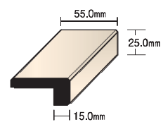
縦用 RC040-21 L=2150mm ¥5,000/本
