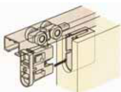
ソフトクローズ機構付上吊引戸用レールセット (2way仕様) RDT-001HR2W(35mm厚ドア用) ¥21,000/セット ※引違戸は2セット必要となります。
