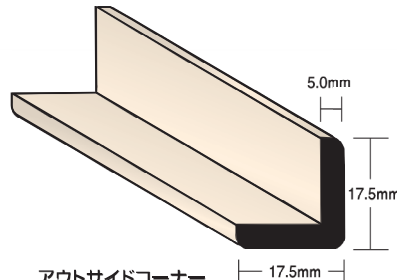
アウトサイドコーナー H3282 ℓ=12'・3660 ㎥ ¥2,800
