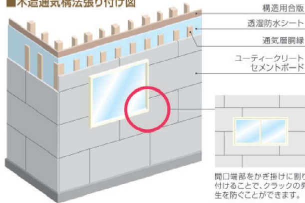
■木造通気構法張り付け図
