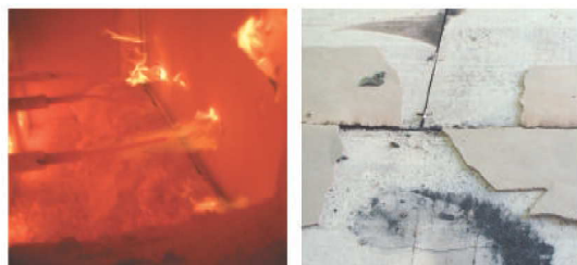
45分準耐火試験状況（左：外壁燃焼時 右：燃焼後）
