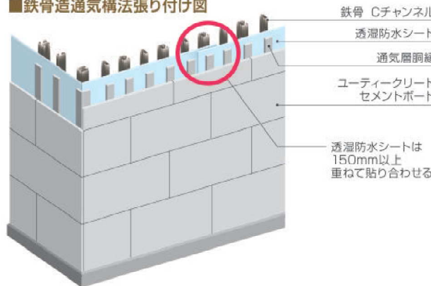
■鉄骨造通気構法張り付け図
