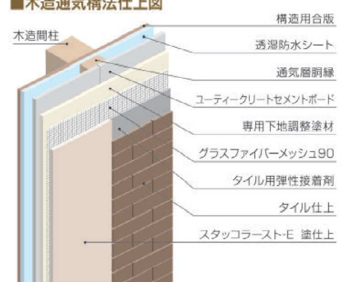
■木造通気構法仕上図
