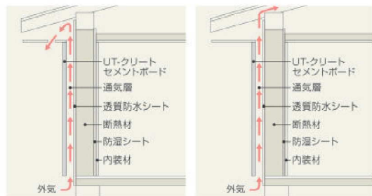
軒天見切縁より排気する構造
