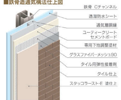
■鉄骨造通気構法仕上図
