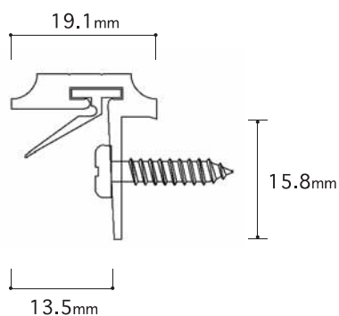
ドアガード
