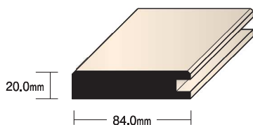
サッシ枠 RC601-39 ℓ = 3900 ㎜ ¥7,700
